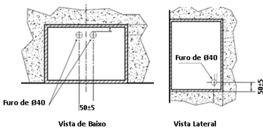
Figura 3 – Localização das zonas circulares para colocação dos bucins
